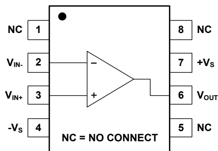
SOIC-8
