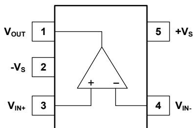
SOT-23-5/SC70-5
